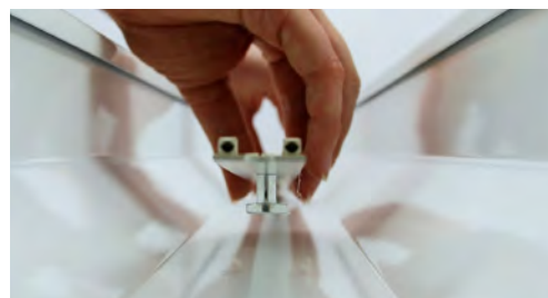
Fixation solide des luminaires grâce à des pieds magnétiques en néodyme amovibles
